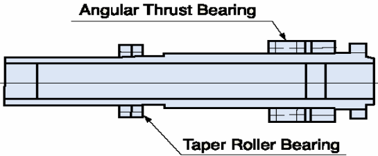
Fig 4: Z340 SM spindle
